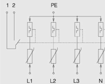
结构图
