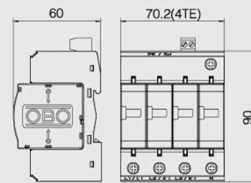
尺寸图
